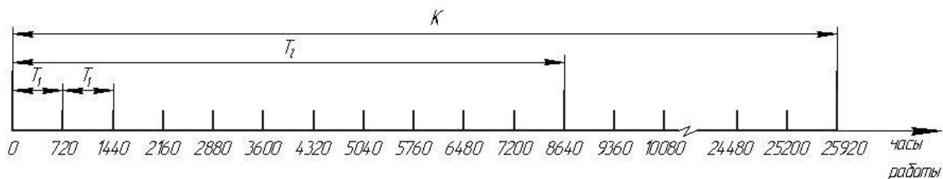
Рисунок 1- Структура ремонтного цикла
